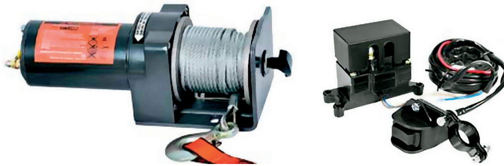
ATV/UTV Vinssi / Winch 907 Kg Kestomagneetti / Permanent magnet 12 V DC
